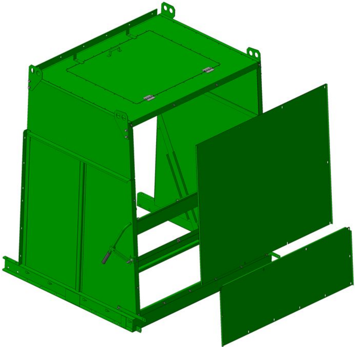
Мал. 2 Капот ПКРБ 271.09.01.00.00.00.00
